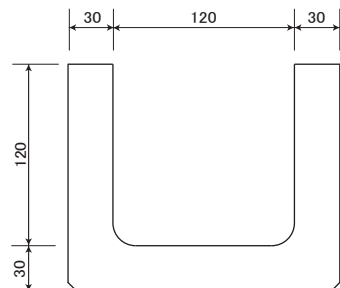
【本体 120】 17kg
