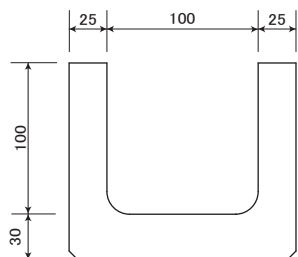
【本体 120】 17kg
