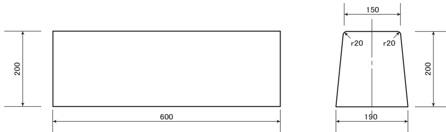
【両面歩車道境界ブロック A】 JIS A 5371 47kg
