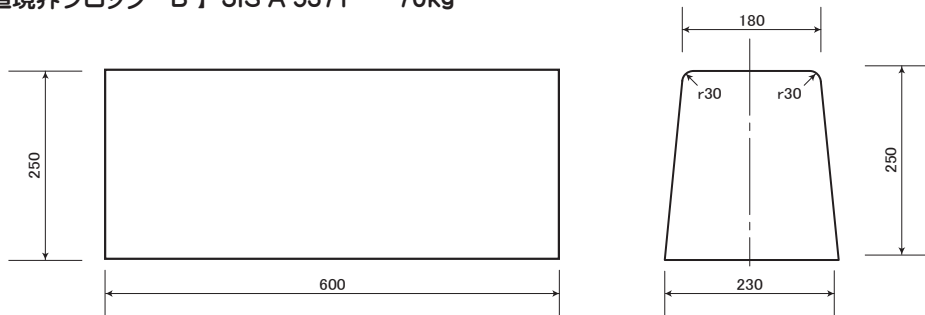
【両面歩車道境界ブロック B】 JIS A 5371 70kg
