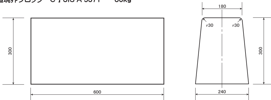
【両面歩車道境界ブロック C】 JIS A 5371 86kg
