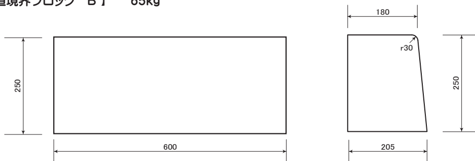
【片面歩車道境界ブロック B】 65kg
