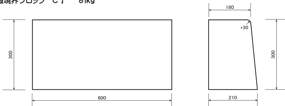
【片面歩車道境界ブロック C】 81kg
