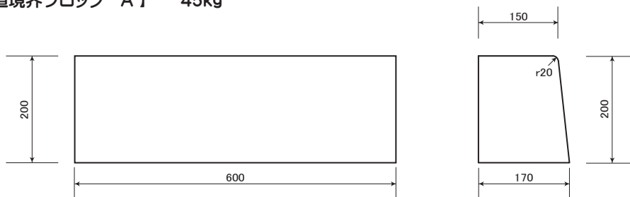
【片面歩車道境界ブロック A】 45kg
