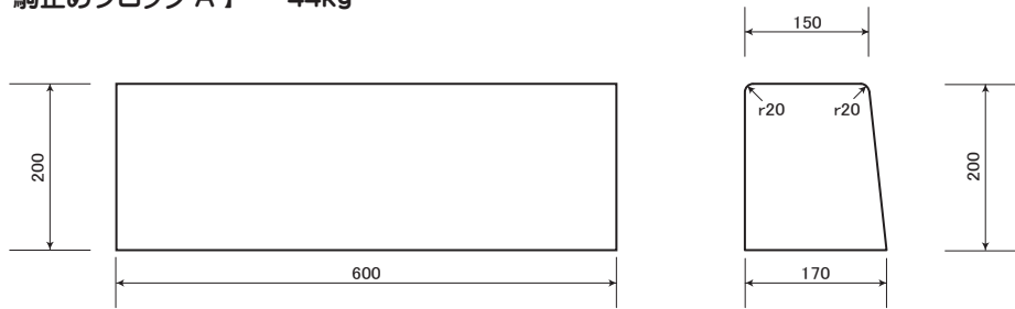
【兵庫県型 駒止めブロック A】 44kg
