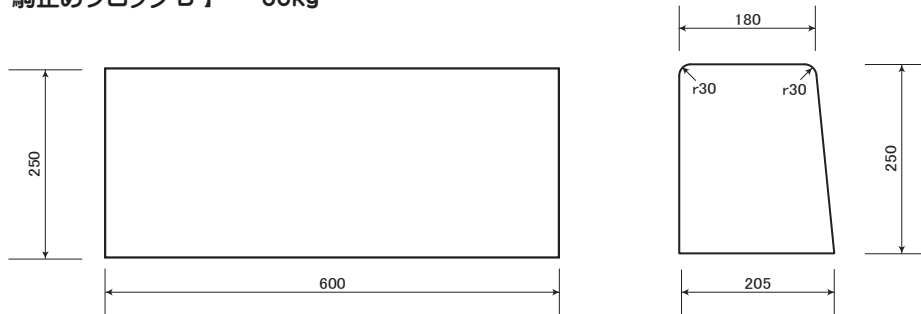
【兵庫県型 駒止めブロック B】 66kg
