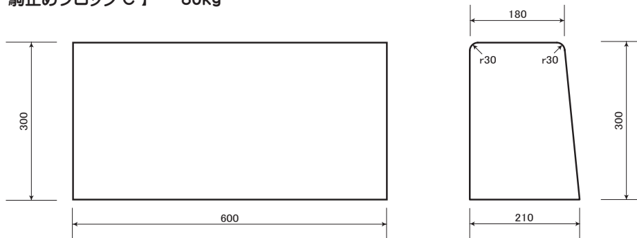
【兵庫県型 駒止めブロック C】 80kg
