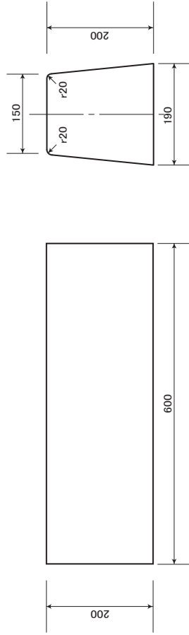
【両面歩車道境界ブロック A】 JIS A 5371 47kg
